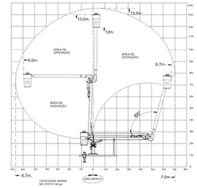
Diagrama Operacional de Cargas e Alcances
